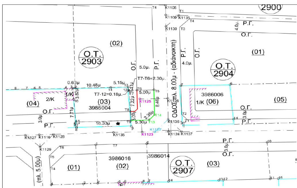
Απόσπασμα του εκπονηθέντος διαγράμματος τροποποίησης
