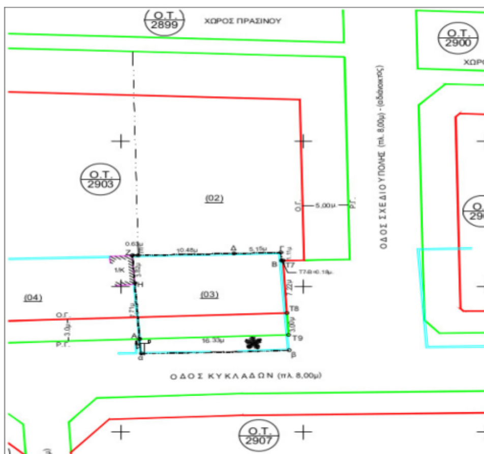
Απόσπασμα του εκπονηθέντος τοπογραφικού διαγράμματος από τον Μάιο 2019
